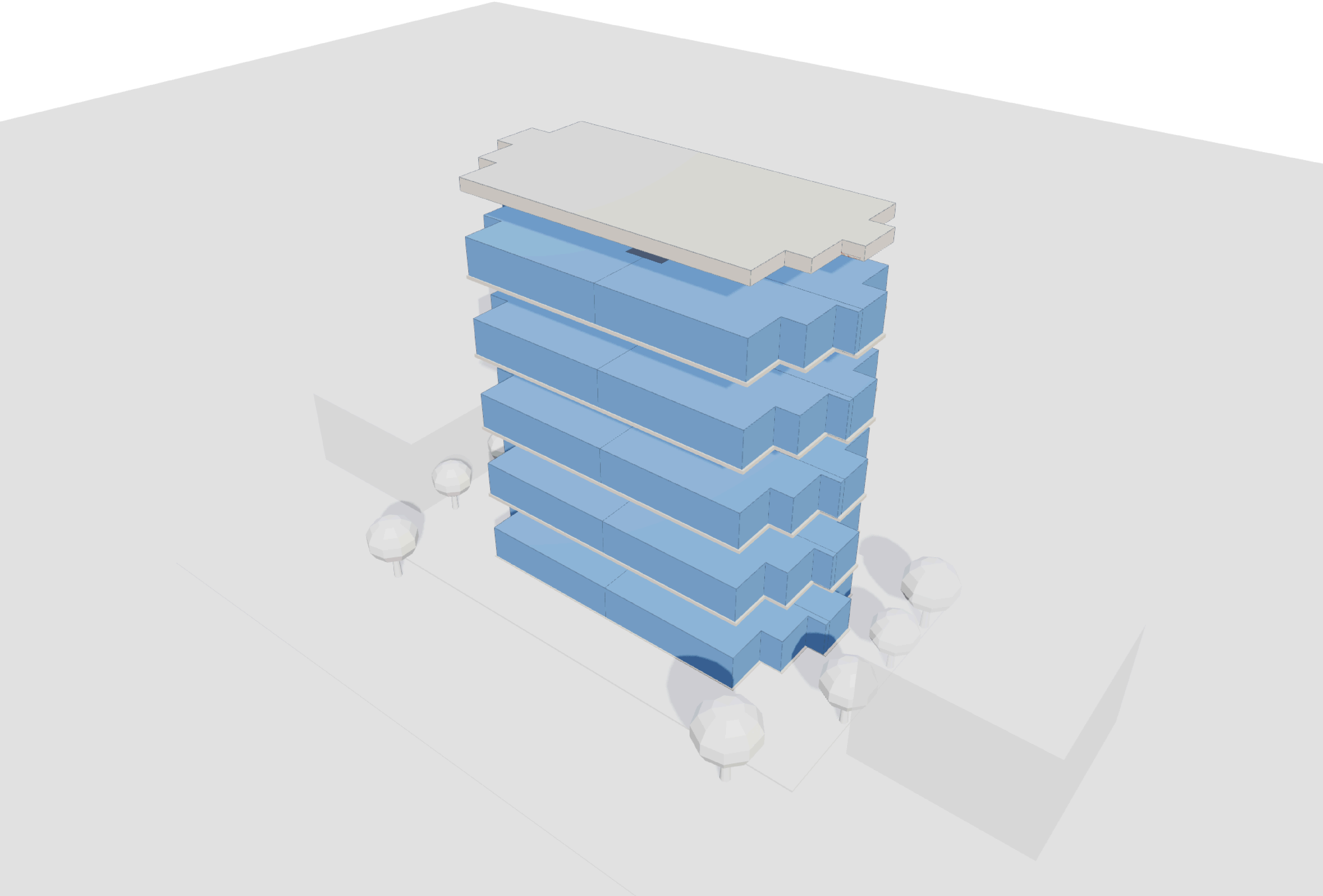
Modelo volumétrico generado desde EL PORTAL.DWG - geometría, cotas y áreas del plano - el modelo muestra el apartamento terminado; el alcance de entrega es el del cuadro correspondiente
